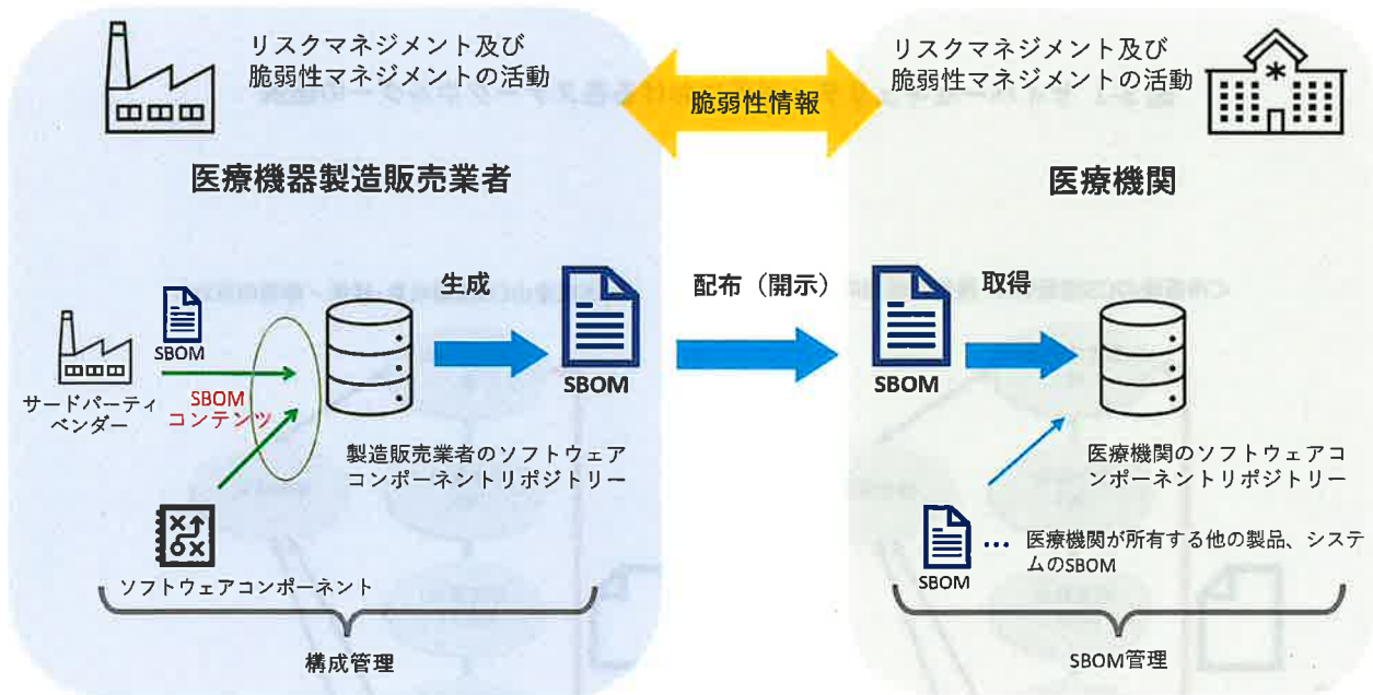
図 4 SBOM の全体的なフレームワーク
